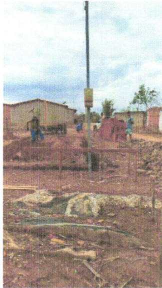
Foto 17 - LOCACAO CONVENCIONAL DE OBRA, UTILIZANDO GABARITO DE TÁBUAS CORRIDAS PONTALETADAS
